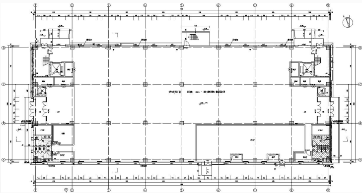
6#首层平面布置
