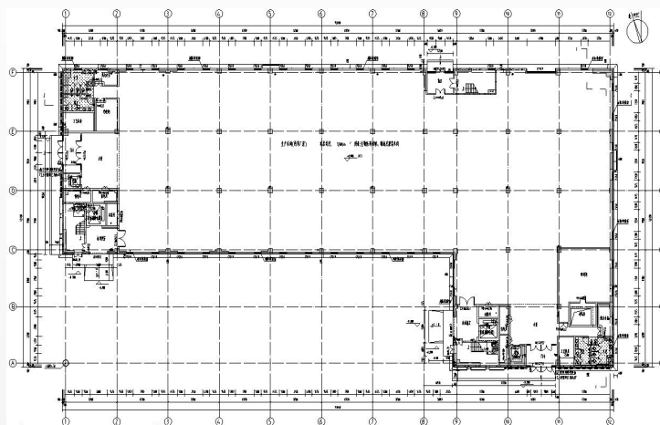
首层平面布置
